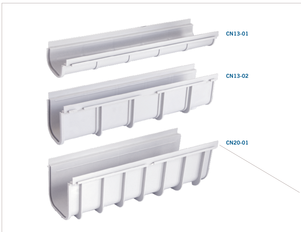
Scarichi inferiori canaletta H14: ø 50 H16: ø 60-75-90
